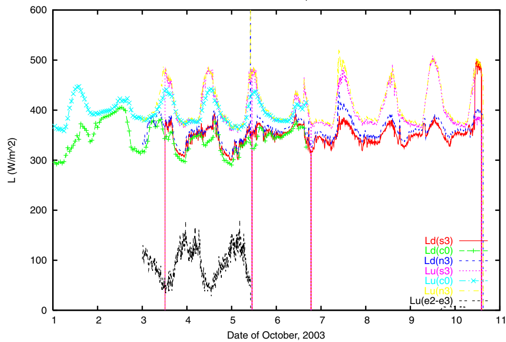
L_down &amp; L_up
