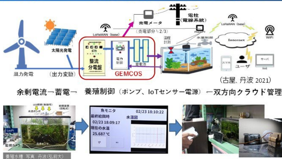
図 2. 余剰電力の蓄電システム(GEMCOS)を IoT 技術で制御するネットワークシステムの構成と、弘前大学で実施した小規模人工養殖モデル実験(2021.1~2)。
