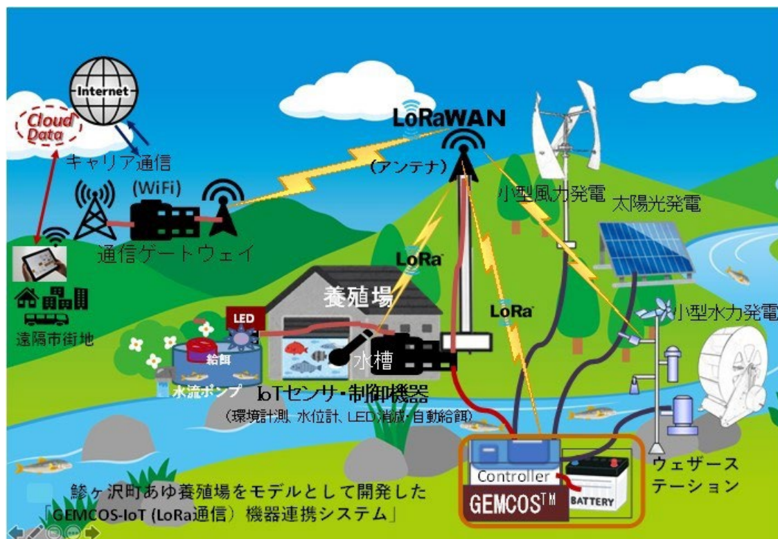
図 3. 青森県鯉ヶ沢町の白神山麓・赤石川流域にあるアユ養殖場で実施した、GEMCOS-IoT システムを活用した設備、LoRa ネットワークシステムの構成および実証試験の概要。
