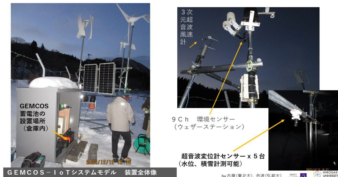
図 4. 鯉ヶ沢町立アユ養殖場で実施した、GEMCOS-IoT システム装置、遠隔的な環境計測 (ウェザーステーション) と機器制御用 GEMCOS 蓄電池、人工養殖モデル実証試験の風景。
