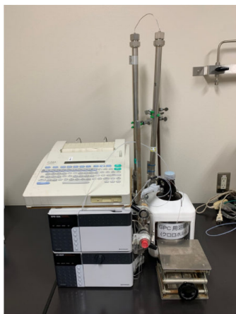
リサイクル分取HPLC [ゲル浸透クロマトグラフ (GPC)]
